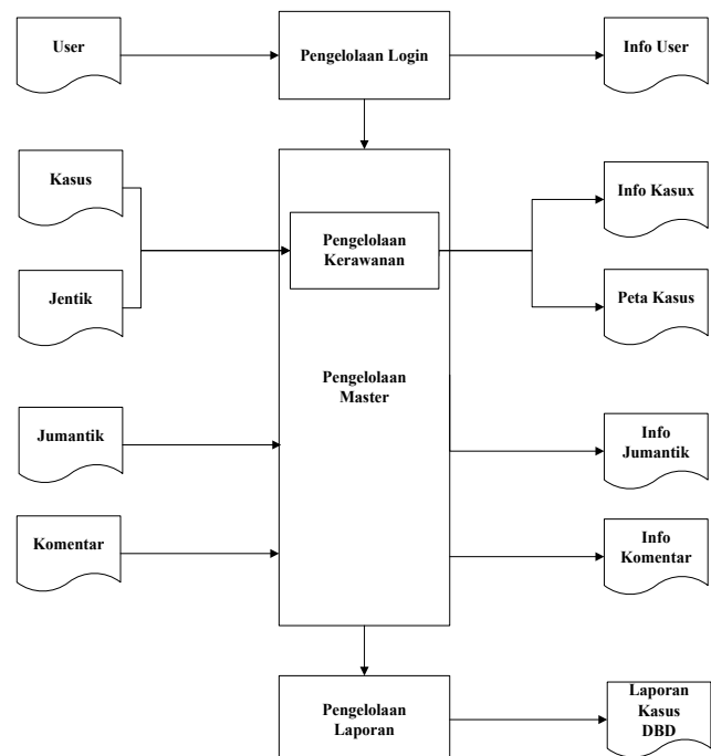
Gambar 3. Arsitektur Perangkat Lunak
