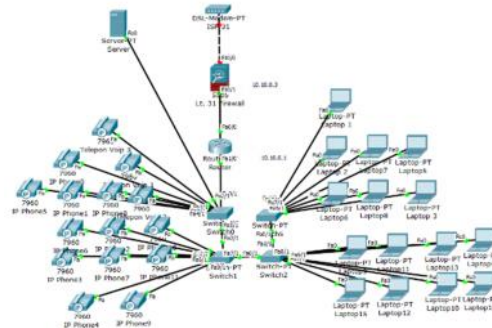
Fig. 1. Rancangan Topologi PT XYZ
