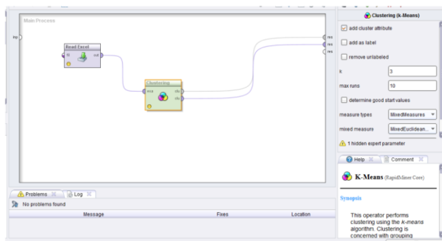
Gambar 1. Algoritma K-Means dengan nilai K = 3
