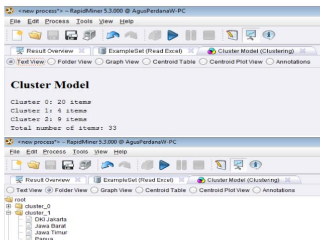
Gambar 2. Hasil Klastering dengan K = 3
