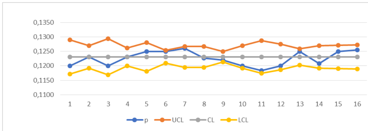
Gambar 2. Peta Kendali Proporsi yang telah disesuaikan pada PT 'X'
