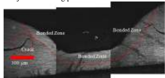
Gambar 18. SS400, dwell time 15 s dan perbesaran 50x.
