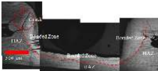
Gambar 14. SPCC, dwell time 30 s dan perbesaran 50x.
