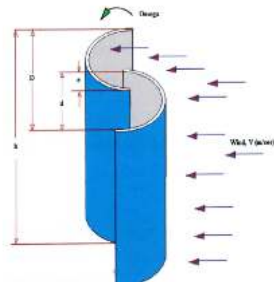
Gambar 1. Savonius Rotor [4].
