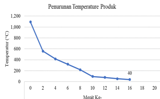
Gambar 4. Penurunan temperatur dengan menggunakan proses pendinginan metode B
